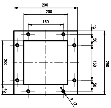
VSTUPNÍ PŘÍRUBA
