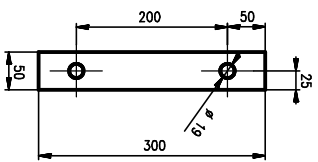
KOTEVNÍ PATKA
