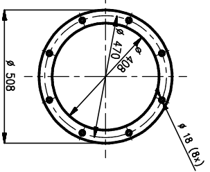
PŘÍRUBA P2
