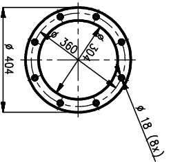
PŘÍRUBA P1
