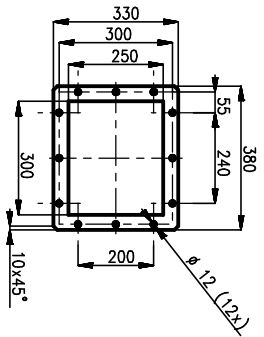
REVIZNÍ OTVOR
